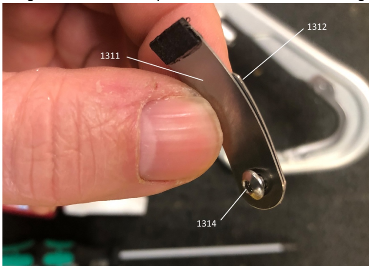
Abbildung 20: Position der Feder-Komponenten hintereinander
