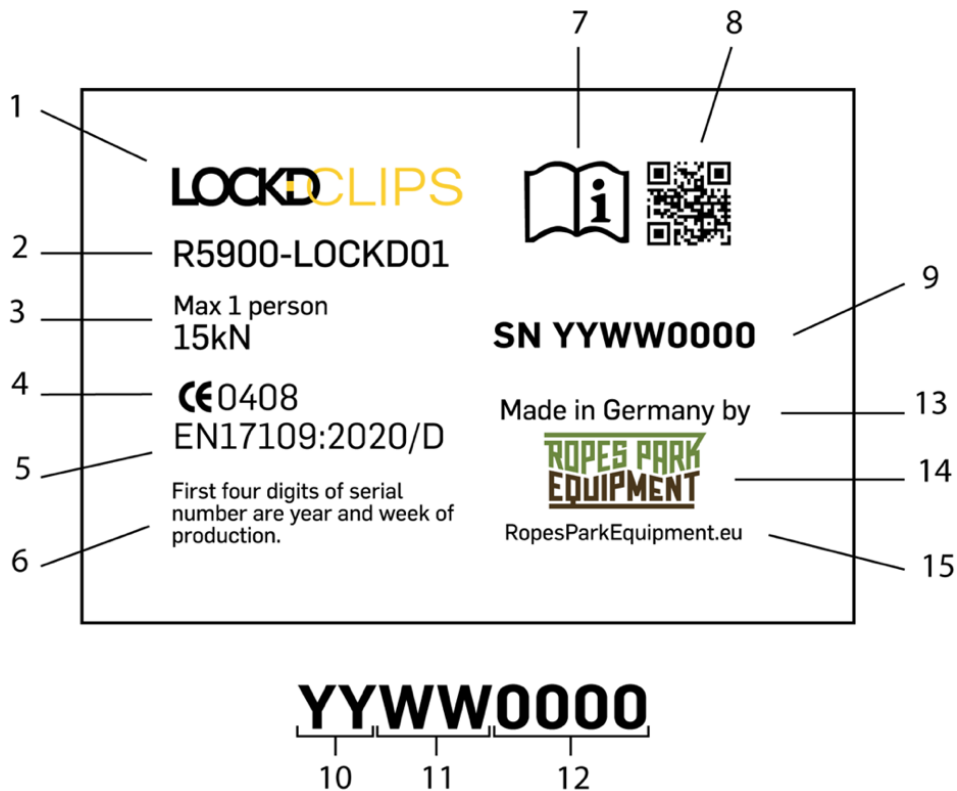
Abbildung 7: Identifikationslabel und Seriennummer
