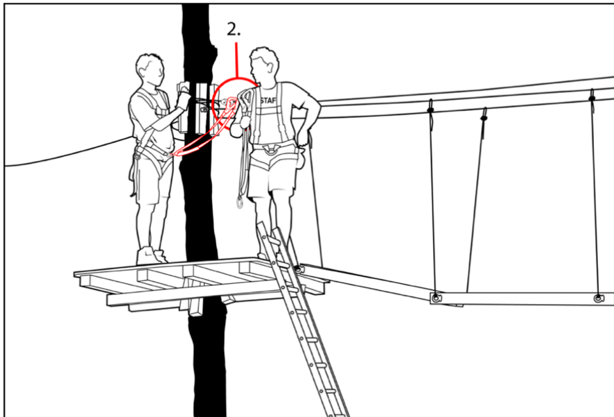
Abbildung 28: Ersatzsystem wird angebracht und Benutzer wird gesichert
