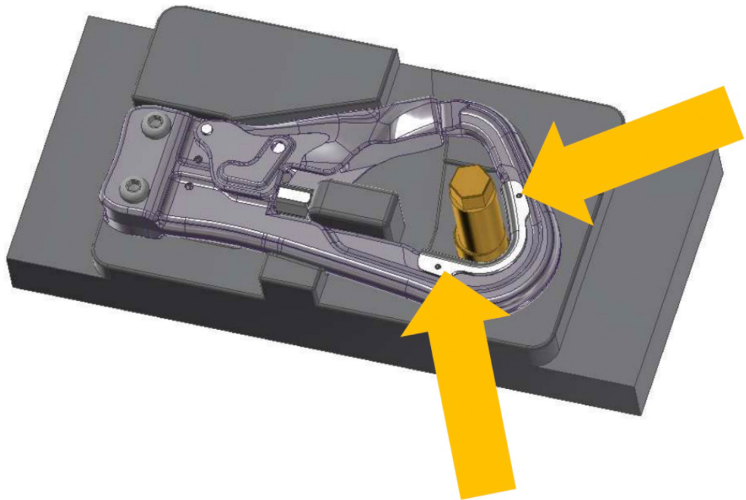
Abbildung 24: Platzieren des Karabinerkörpers im Montageblock
