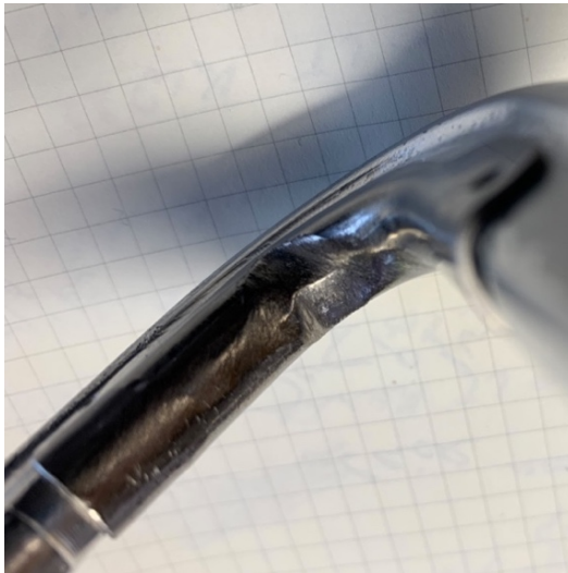
Abbildung 22: Leicht abgenutztes Abriebblech – muss nicht erneuert werden
