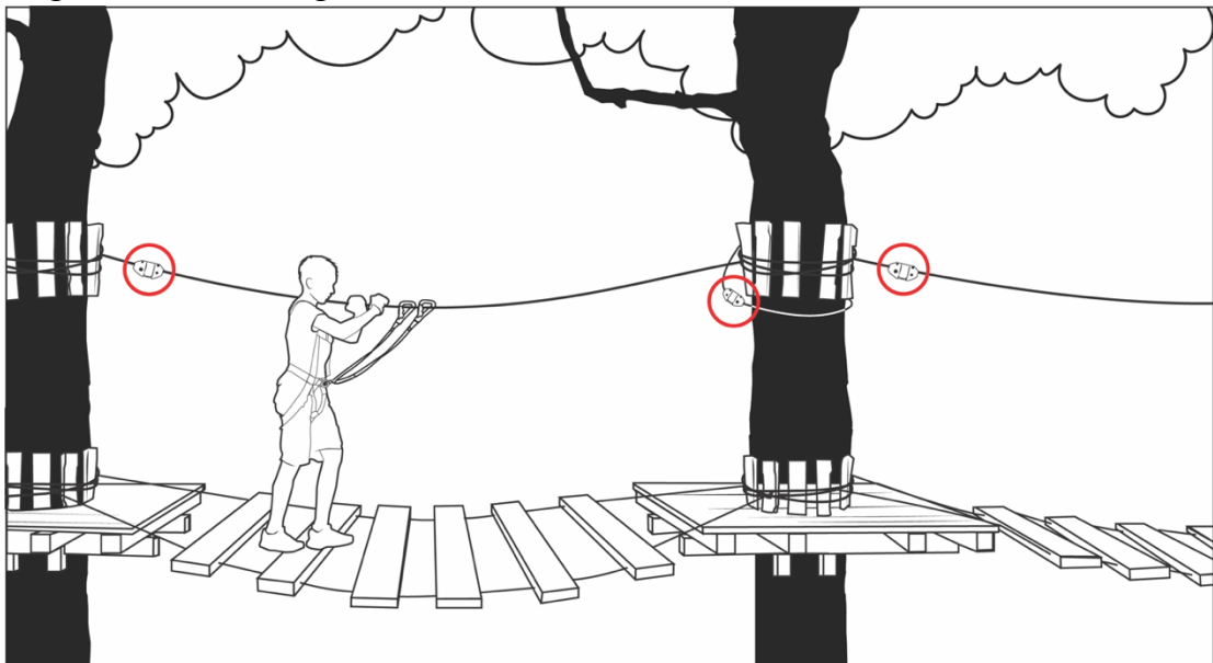
Abbildung 18: Ausstattung eines Parcours mit Tweezlen
