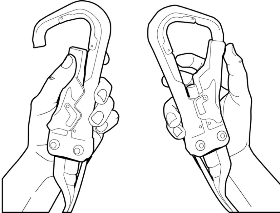
Abbildung 16: Öffnen des Hakens durch Druck auf den Schnapper
