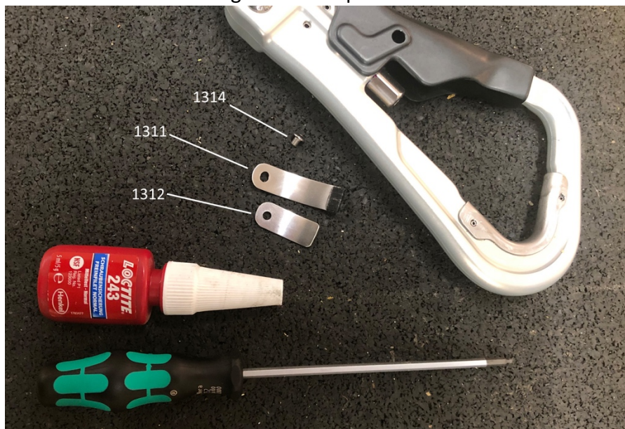
Abbildung 19: Komponenten der Feder des Schnappers
